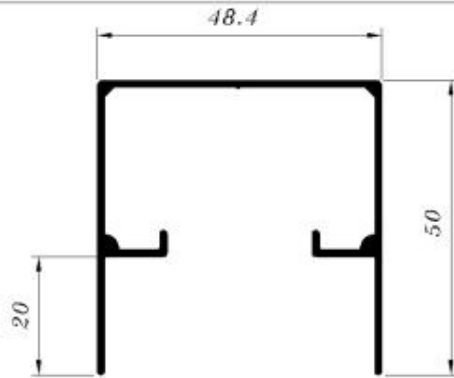
U-397 0.856 kg/m
