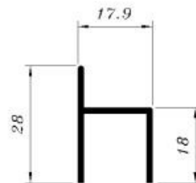
Y-107 0.280 kg/m
