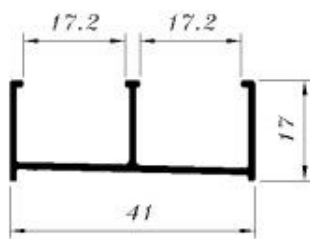
E-117 0.367 kg/m
