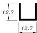
AL-30 0.151 kg/m
