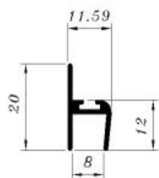
AL-63 0.168 kg/m
